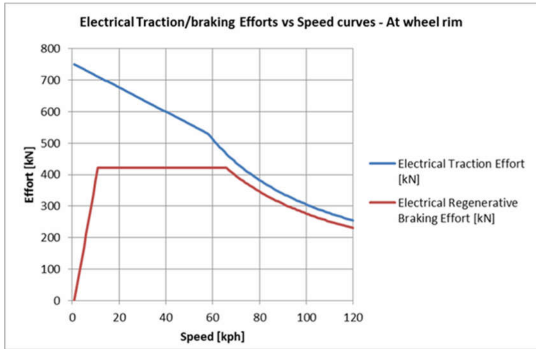
Рисунок 1 – Кривая силы тяги и торможения от скорости на ободе колеса
